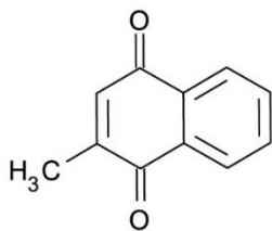
1. Vitamin K3 (Menadione)
