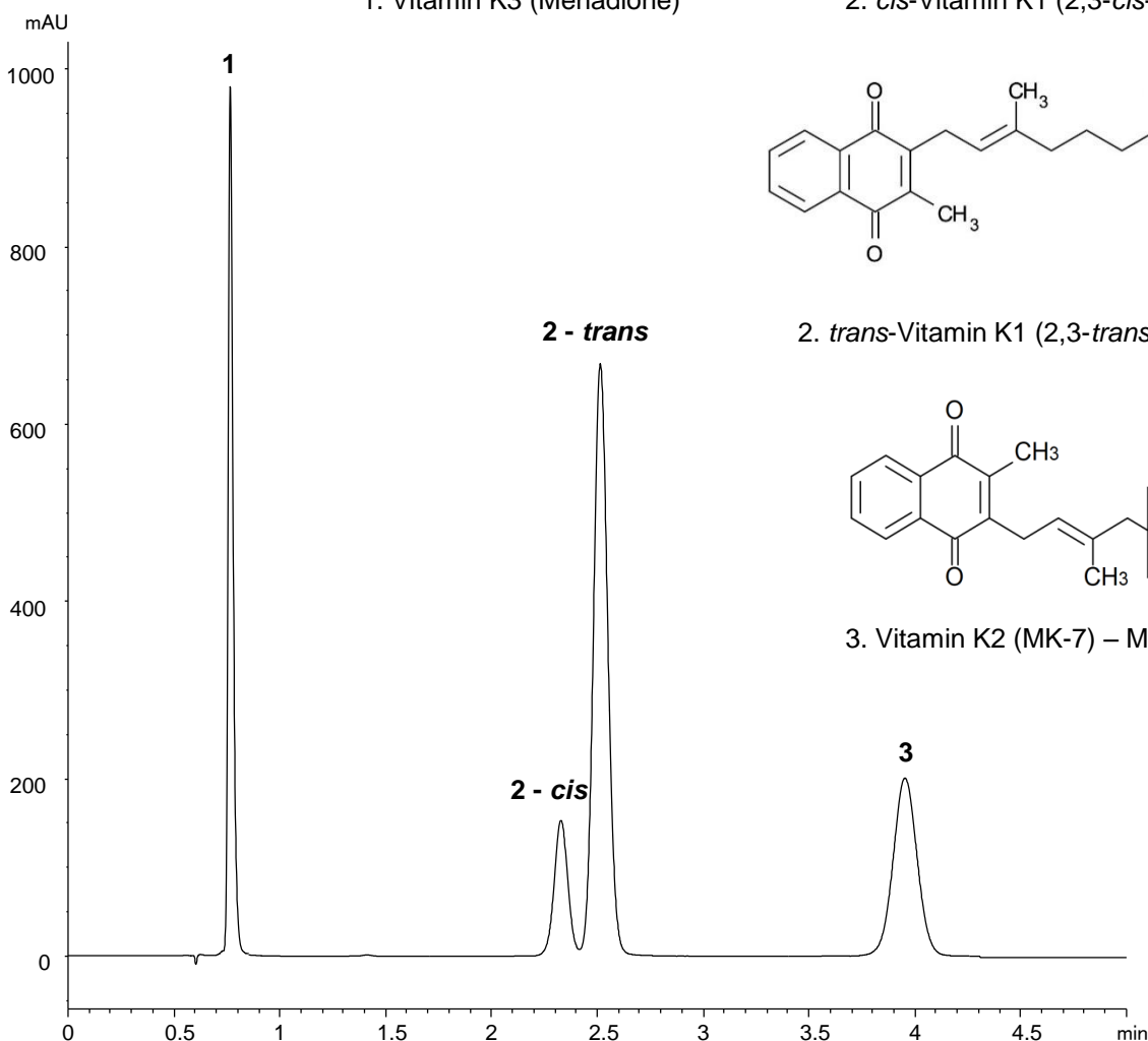
1. Vitamin K3 (Menadione)
