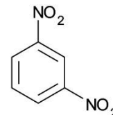
3. 1,3-Dinitrobenzene
