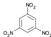
1. 1,3,5-Trinitrobenzene
