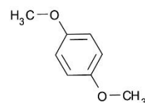
4. 1,4-Dimethoxybenzene
