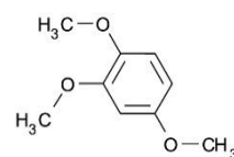
3. 1,2,4-Trimethoxybenzene
