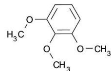
1. 1,2,3-Trimethoxybenzene
