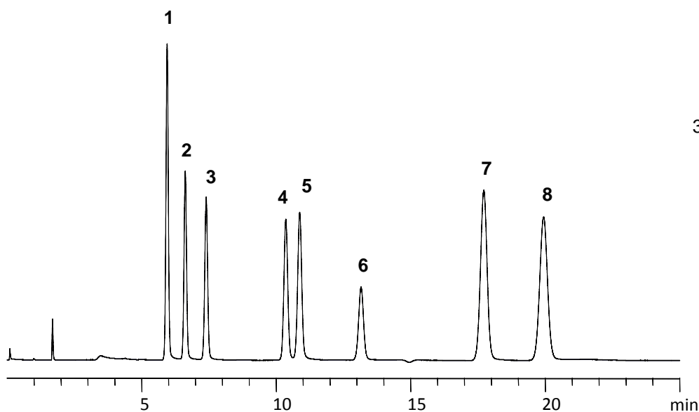
4. 1,4-Dimethoxybenzene
