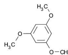
7. 1,3,5-Trimethoxybenzene
