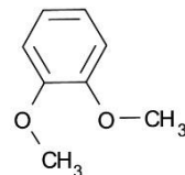
2. 1,2-Dimethoxybenzene
