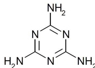
3. Melamine
