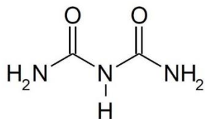
1. Biuret
