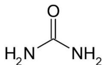
2. Urea
